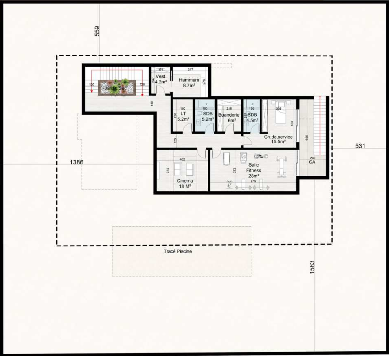
Plan Sous-sol - Villa Type A 1
